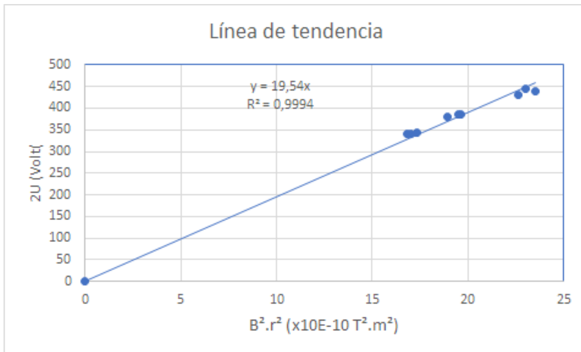
Gráfico 1: Representación gráfica de 2U (en Volts) en función de B^2.r^2 (en \times 10E-10 T^2.m^2 ).
